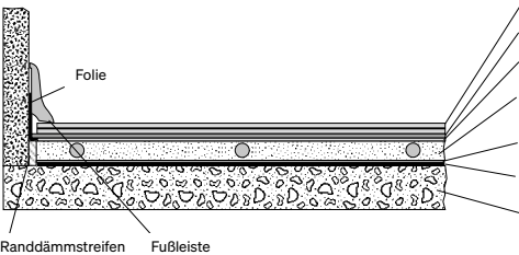
Aufbau der schwimmenden Verlegung
