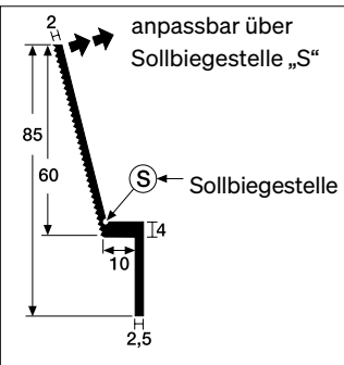
Schrägwinkel 3402 Mit umlaufenden Kleberillen, Aluminium, naturfarbig, mit versenkten Bohrungen, Holzschrauben mit Kreuzschlitz 3,5 Ø × 20 mm liegen bei. Härte: ca. 75 N/mm². Länge: 100 cm
